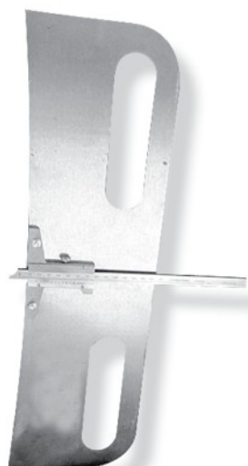
Dispositif de mesure usure des plateaux r 1500 mm - 261.811 r 2750 mm - 261.812
