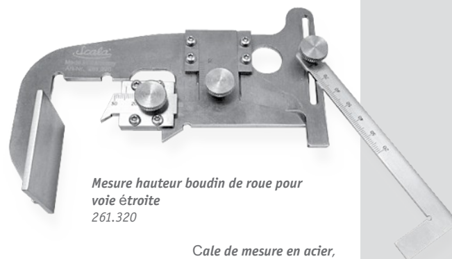
Pied à coulisse à pointes compas pour mesure longueurs et diagonales sur châssis et bogies 20 - 2000 mm - 608.320 20 - 4000 mm - 608.340
